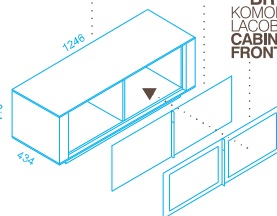
BR 36 KOMODA Z FRONTEM PRZESUWNYM Z PŁYTY LAMINOWANEJ CABINET WITH SLIDING, LAMINATED BOARD FRONT
