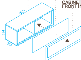
BR 34 KOMODA Z FRONTEM Z PŁYTY LAMINOWANEJ CABINET WITH LAMINATED BOARD FRONT
